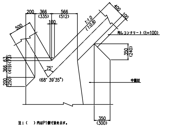
"b"部詳細図 縮尺1:20
