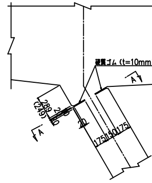
"a"部詳細図 縮尺1:20
